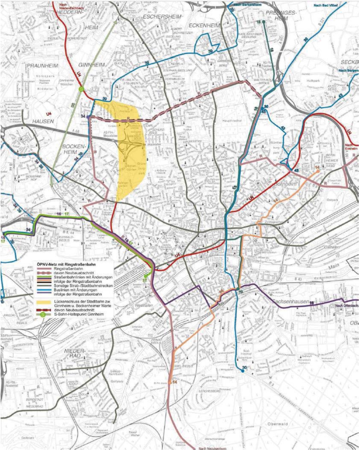
Abbildung 2: Liniennetz des Langfrist-Szenarios mit integriertem Kurzfrist-Szenario
