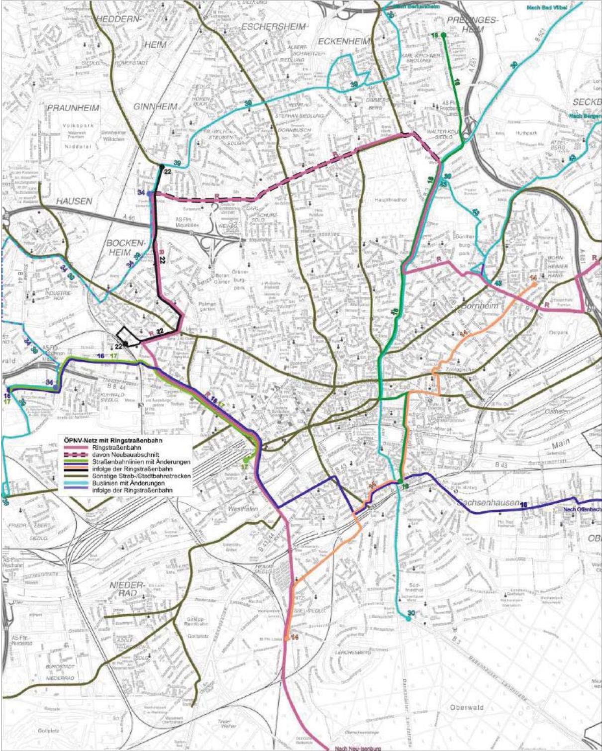
Abbildung 1: Liniennetz des Kurzfrist-Szenario: Linie RING (R) und durch sie veränderte Straßenbahn- und Buslinien
